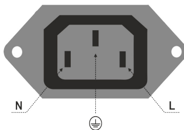
ZÁSUVKY V OVLADAČI
